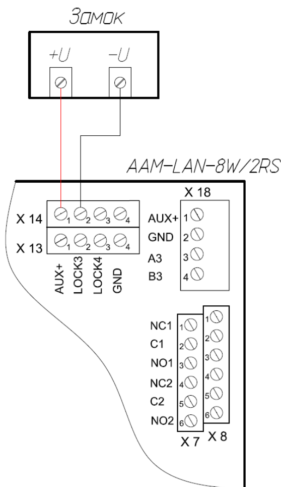
Рисунок 17. Пример подключения замка к токовым ключам.
