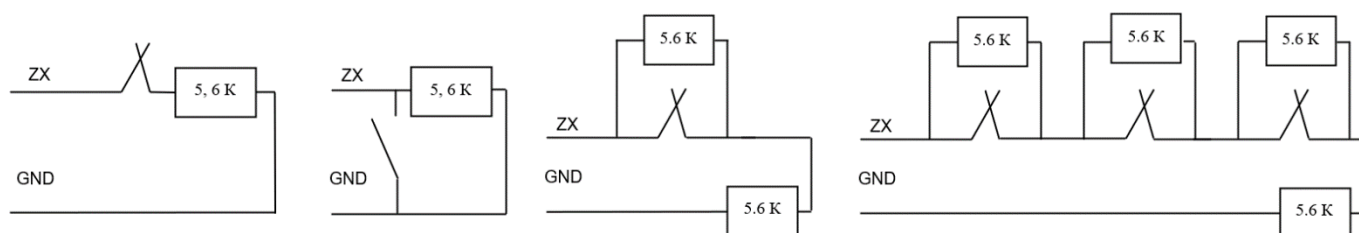
Рисунок 13. Пример подключения охранных датчиков с выключенным контролем целостности линии.
