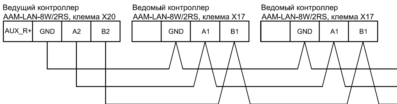
Рисунок 1. Подключение ведомых ААМ-LAN-8W/2RS к ведущему ААМ-LAN-8W/2RS.
